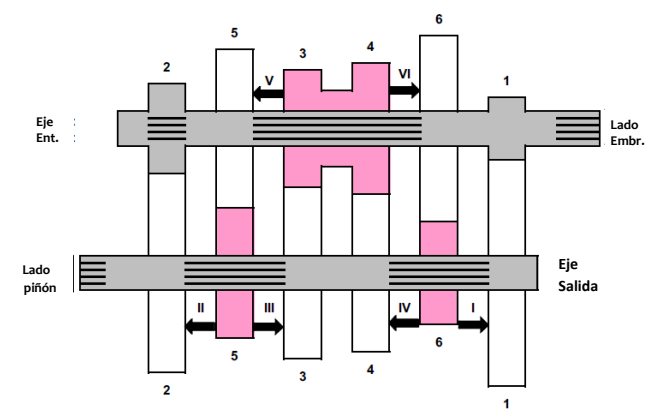
Resumen. Caja de cambio de Caja de 6 Velocidades Pulsar 200
