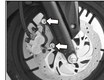
Montaje de caliper delantero
