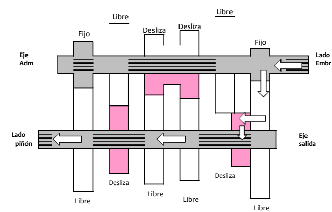
Flujo de la Potencia en 1ª
