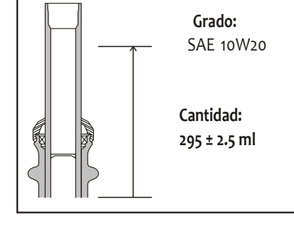
Grado y Capacidad de Aceite de Horquilla Frontal
