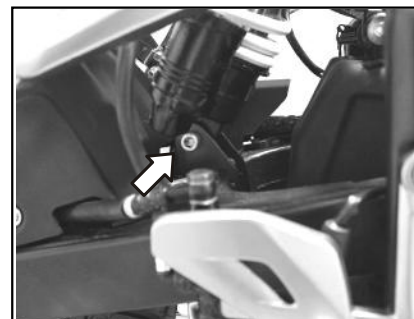
Perno inferior de mono shock
