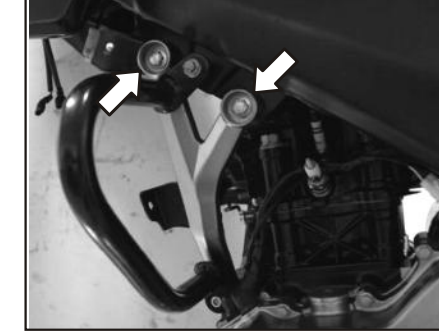
Pernos Superiores lado IZQ. del Motor
