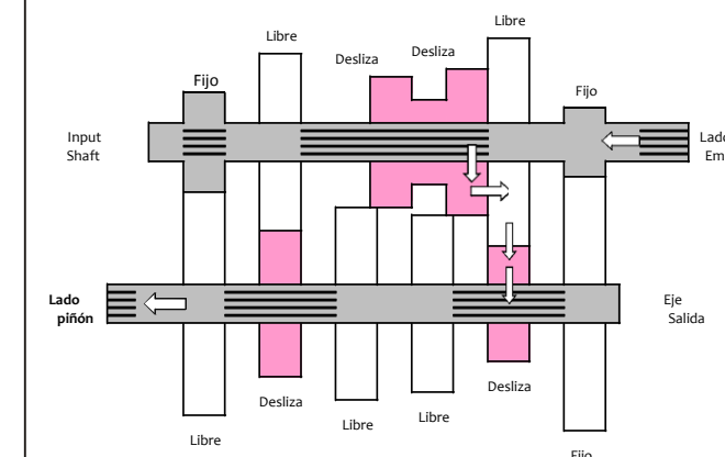
Flujo de la Potencia en 6ª
