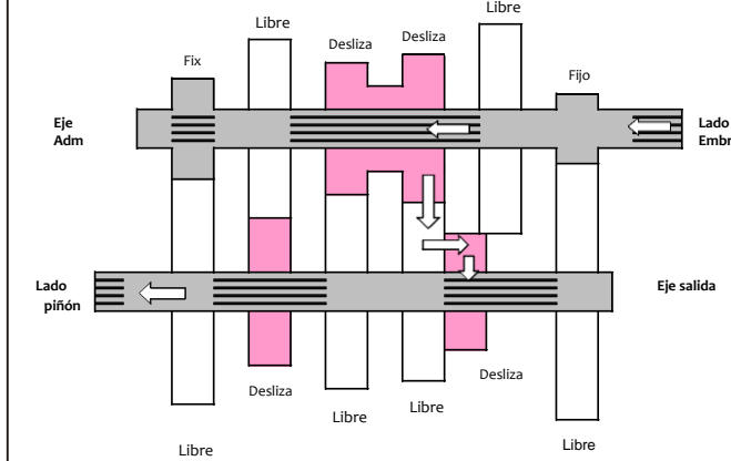
Flujo de la Potencia en 4ª
