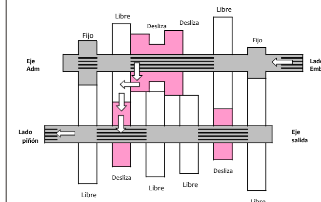
Flujo de la Potencia en 5ª
