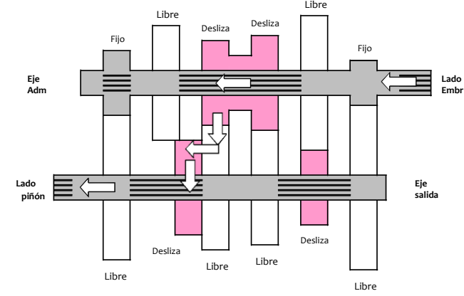
Flujo de la Potencia en 3ª
