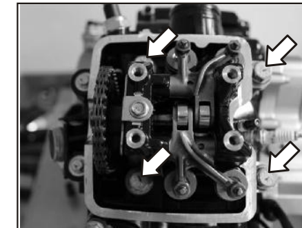
Pernos Grandes de la Culata
