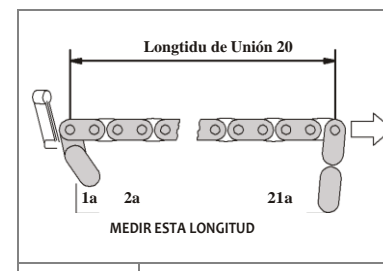
Longitud de Cadena de Leva
