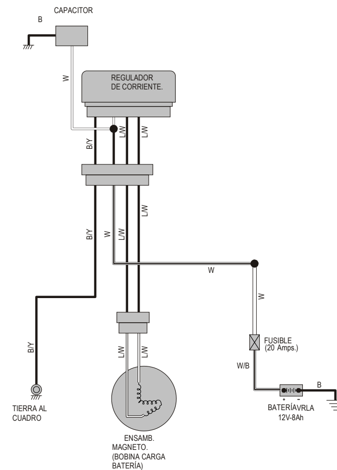
Circuito de Carga de Batería
