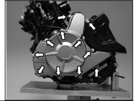
Pernos de Cubierta de Magneto
