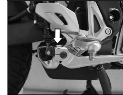
Perno del pedal del freno trasero
