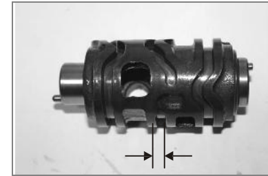
Grosor Ranura de Tambor de Cambios
