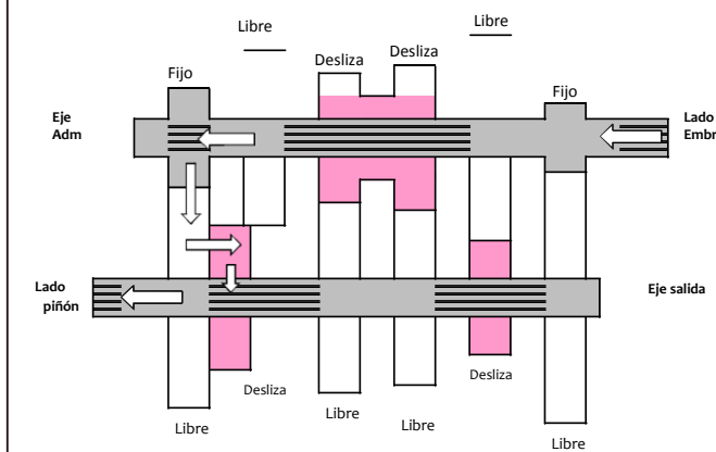
Flujo de la Potencia en 2ª
