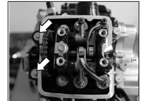
Pernos Pequeños de la Culata
