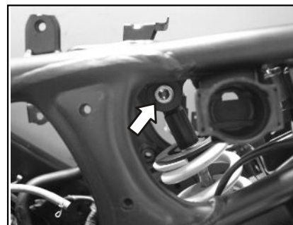
Perno superior de mono shock
