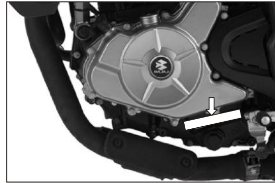
Ubicación del Número de Motor En el lado izquierdo del Cárter Cerca al Pedal de Cambio (Código alfanumérico de 11 dígitos)
