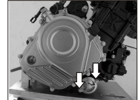
Perno de Cubierta de Filtro de Aceite
