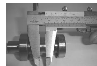
Grosor de Leva
