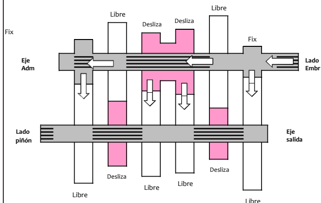
Flujo de la Potencia en la Posición Neutro
